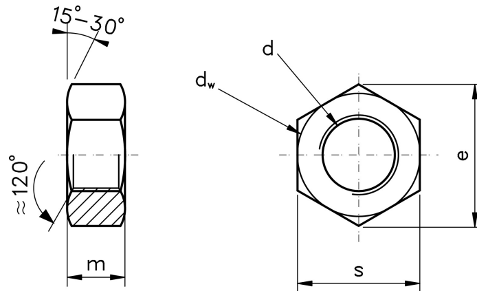
Figure 1: DIN 934 Metric Full Hex Nut
